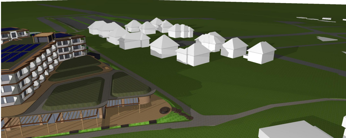
Sonnenstudie 21/12 13:00
