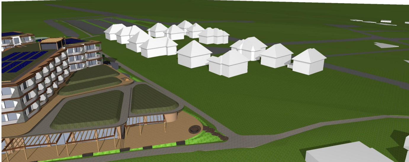
Sonnenstudie 21/03 10:00
