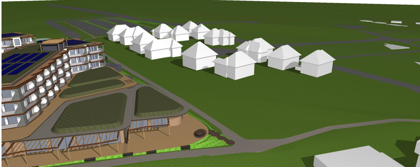
Sonnenstudie 21/06 08:00
