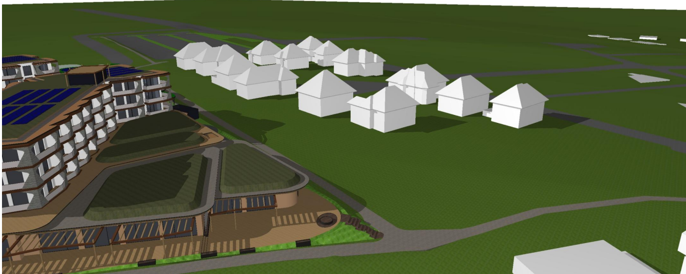
Sonnenstudie 21/03 15:00
